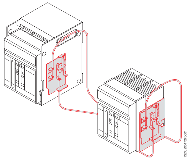
Horizontal interlock
